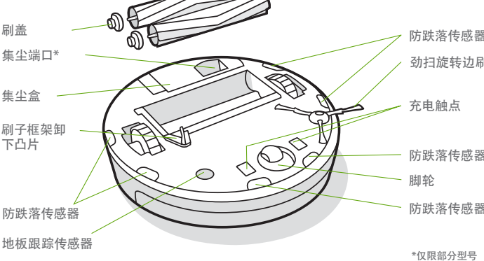
底视图
